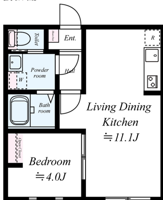
【間取り図】
